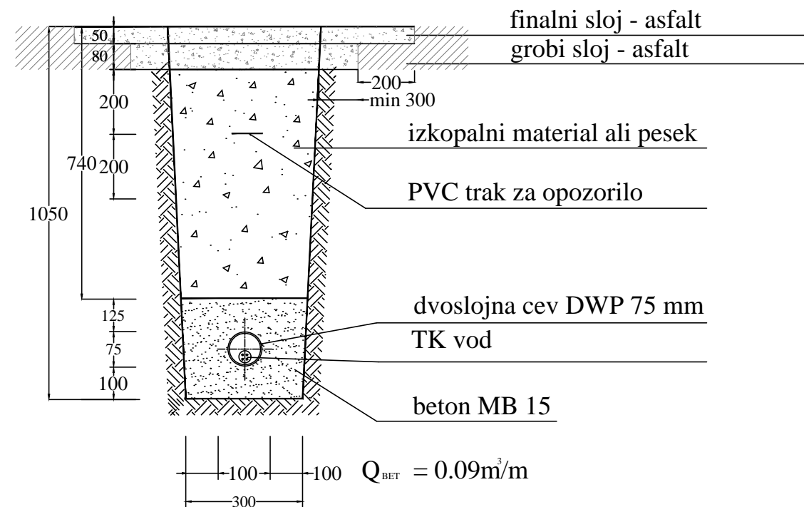
kabelska kanalizacija - 1 cev DWP 75 mm
